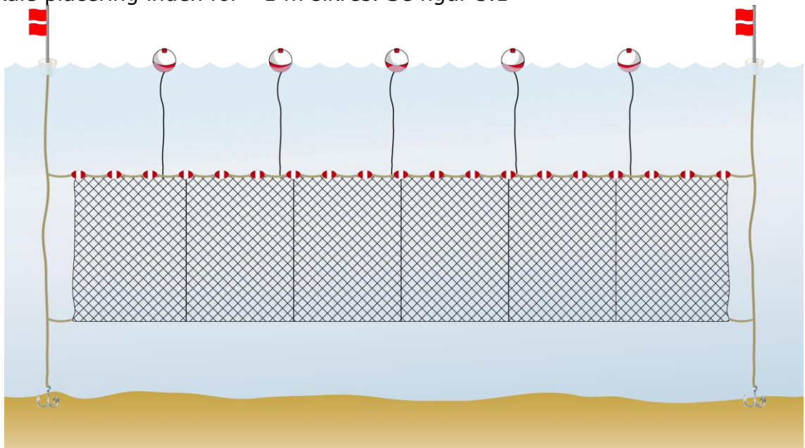
Figur 5.1 Skematisk tegning af opsætning af pelagisk gællegarn. OBS – for beskrivelse af antallet af og fordelingen af netsektioner og maskestørrelse – se tekst.
