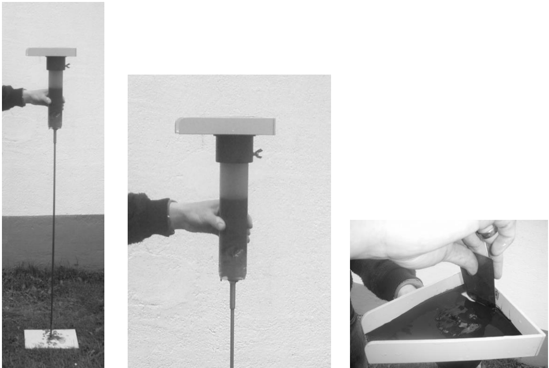
Figur 7.2 Opstilling til afskæring af overfladesegment.
