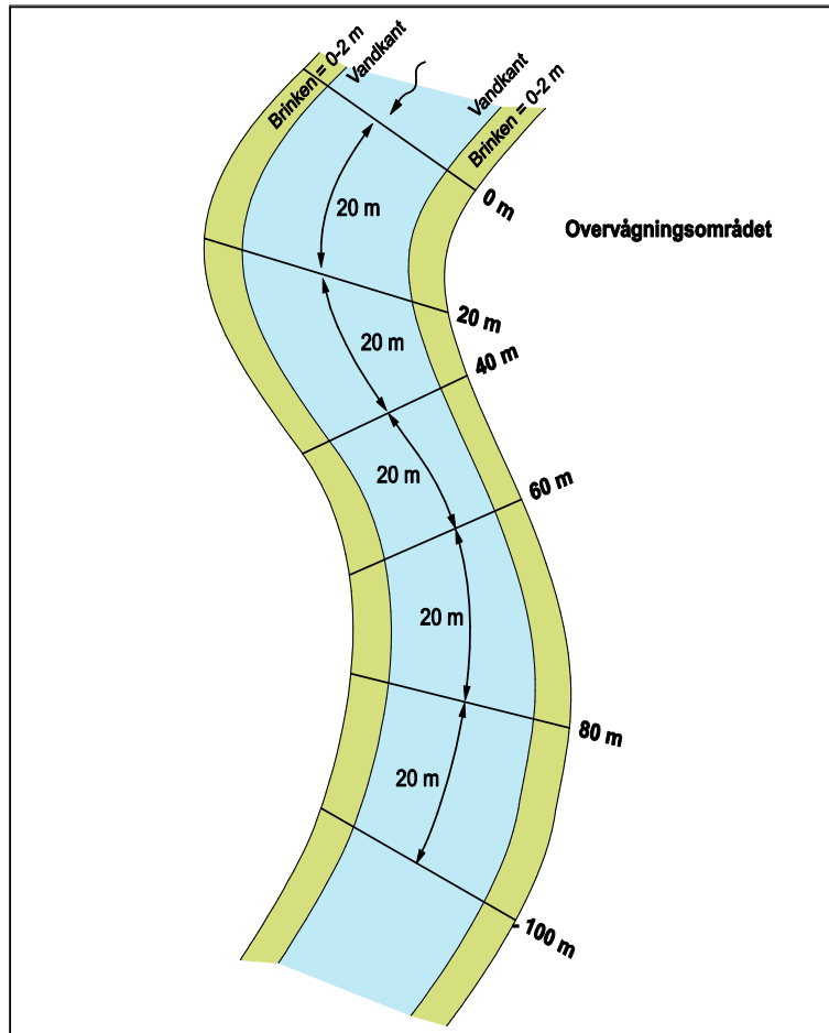
Figur 1. Stationsopsætning, anvisning på udlægning af transekter. OBS: Den viste 0-2 m brink indgår IKKE i NOVANA programmet efter 2007.
