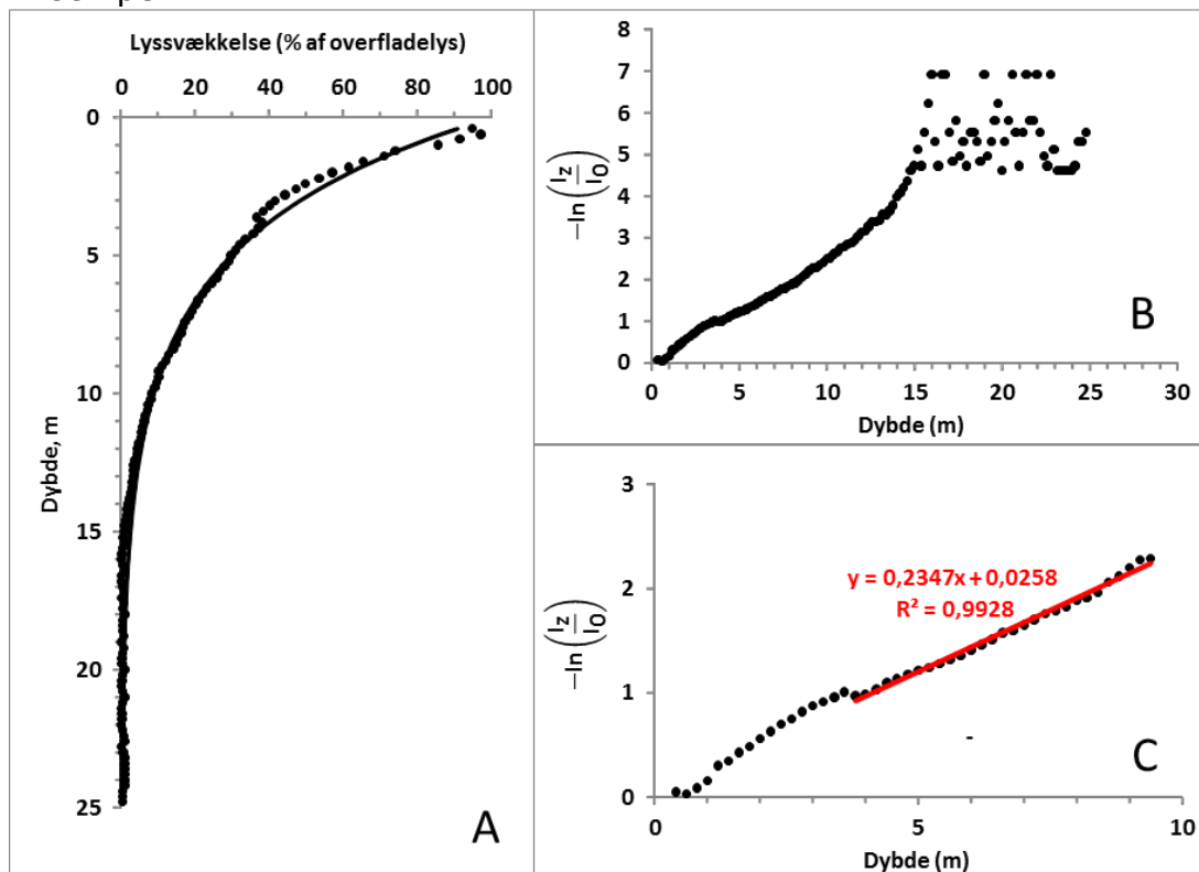
Fig. 5. Lyssvækkelseskurve (A) og den logaritmetransformerede lyssvækkelse (B og C) vist mod vanddybden. A: Lyssvækkelsen (i % af overfladelys) på 25 m's vanddybde målt mellem 0,2 m og 24,8 m i 0,2 m intervaller (sorte punkter). Den beregnede lyssvækkelse beregnet fra K_d er vist ved den fuldt optrukne linje. B: Lyssvækkelseskurven på Fig. A logaritmetransformeret. C: Lyssvækkelseskurven på Fig. A logaritmetransformeret i intervallet 0,2 - 9,8 m. Den røde regressionsline er beregnet for intervallet 3,8 - 9,4 m og resulterer i K_d = 0,2347 \text{ m}^{-1} .
