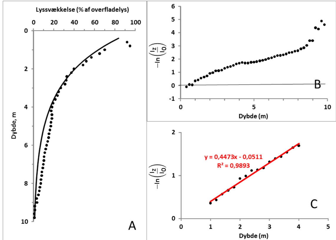
Fig. 6. Lyssvækkelseskurve (A) og den logaritmetransformerede lyssvækkelse (B og C) vist mod vanddybden. A: Lyssvækkelsen ( i % af overfladelyset) på 10 m's vanddybde målt mellem 0,2 m og 9,8 m i 0,2 m intervaller (sorte punkter). Den beregnede lyssvækkelse beregnet fra K_d er vist ved den fuldt optrukne linje. B: Lyssvækkelseskurven på Fig. A logaritmetransformeret. C: Lyssvækkelseskurven på Fig. A logaritmetransformeret i intervallet 1,0 – 4,0 m, hvor den røde regressionsline resulterer i K_d = 0,4473 \text{ m}^{-1} .
