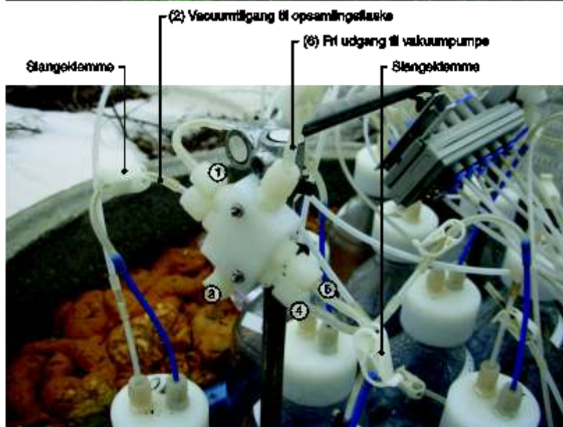
b. 6-vejskobling til vakuum
