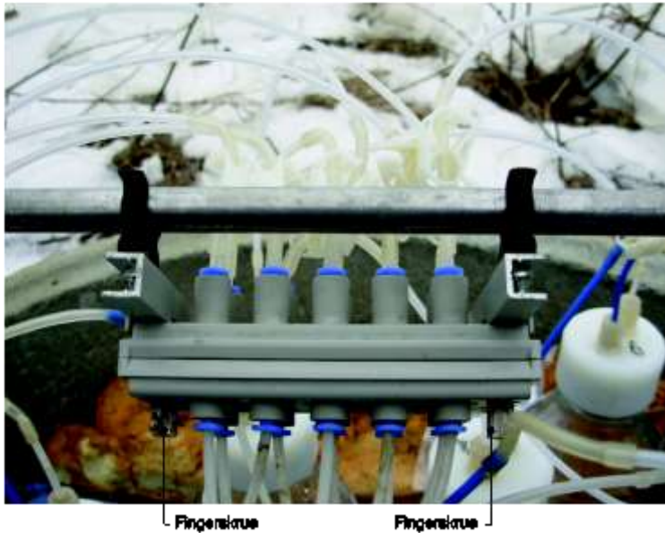
c. Samlet 10-vejskobling.
